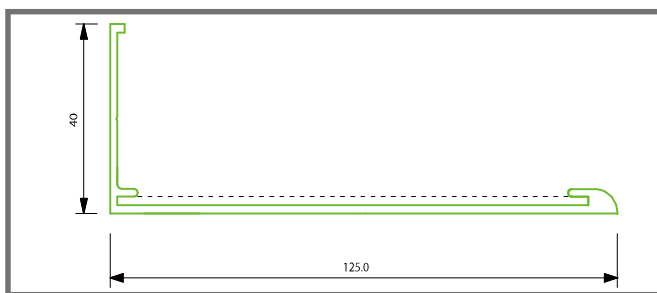
壁側オス材(P06WM)
